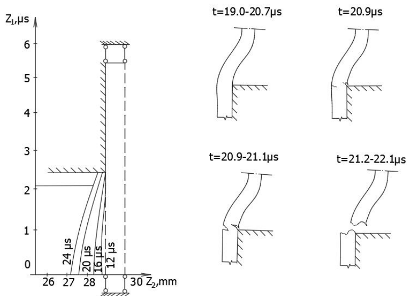
Fig. 9. Crimping
