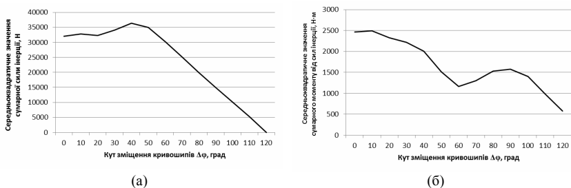
Рис. 6. Графіки зміни середньоквадратичних значень сил інерції \bar{F}_{ic} (а) та моментів від сил інерції \bar{M}_i (б) в залежності від кута зміщення кривошипів \Delta\phi
