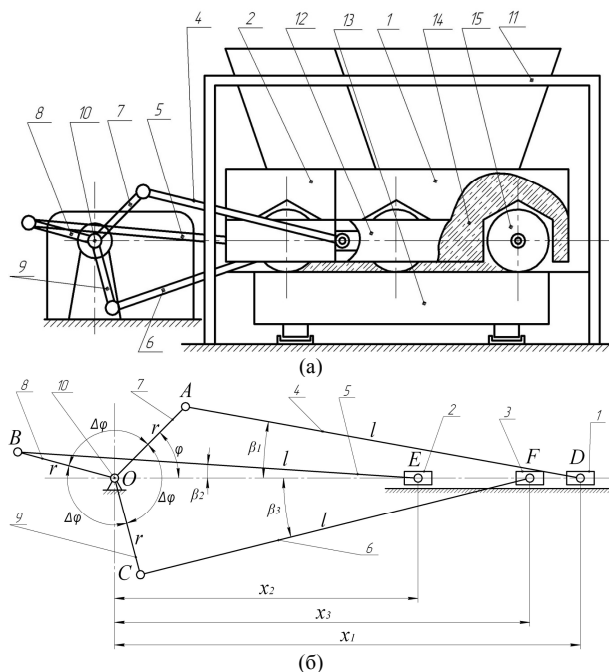
Рис. 1. Роликова формувальна установка з енергетично рівноваженим приводом (а) та її кінематична схема (б)
