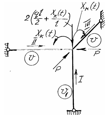
Рис. 5. Розрахункова схема МСЕ
