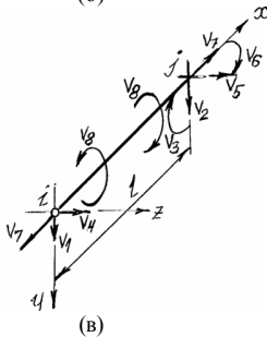
Рис. 3. До прикладу: (а) - розрахункова схема; (б) - основна система методу переміщень; (в) - скінченний елемент
