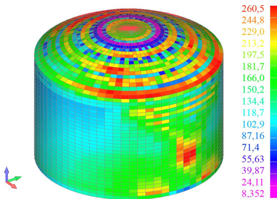
Рис. 4. Загальні напруження паливного резервуару по Мізесу в МПа після оптимізації з жорсткою сегментною оболонкою покриття
