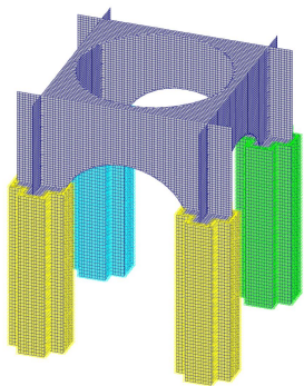
Рис. 8. Об'єднання переміщень всіх вузлів на площинах контакту шару тинькування та цегляних стовпів
