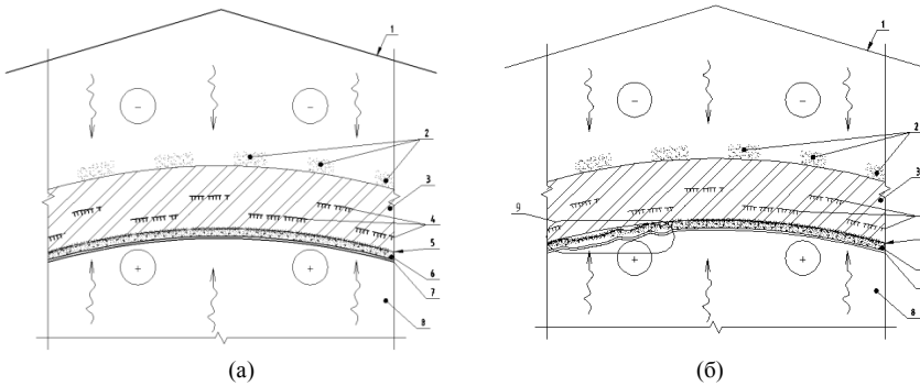
Рис. 7. а,б. Схема складу перекриття горішнього поверху
