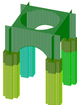
Рис. 9. Моделювання відшарування тинькування (об'єднання переміщень 75% вузлів на площинах контакту шару тинькування та цегляних стовпів)
