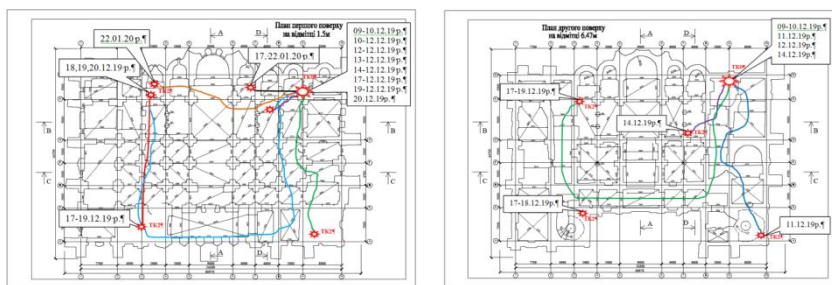
Рис. 3. Місця вимірювання вібрацій в Соборі на відм. +1.5, +6.47м та реєстрація вимірювань в часі (кольоровими лініями показані кабельні мережі між станціями)
