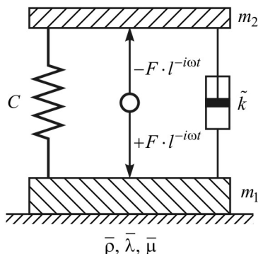
Рис. 1. Геометрія задачі об'ємного ущільнення бетонної/будівельної суміші
