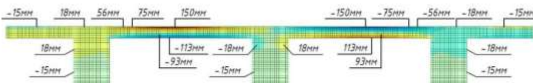
Рис. 11. Переміщення по горизонтальній осі U_x
