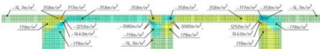
Рис. 10. Ізоліїнї дотичних напружень \tau_{xy}
