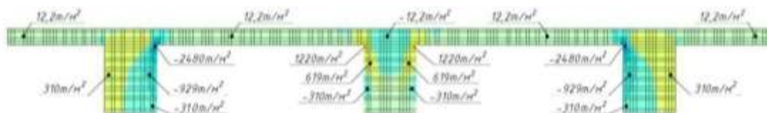
Рис. 8. Ізоліїнї нормальних напружень \sigma_{xx}
