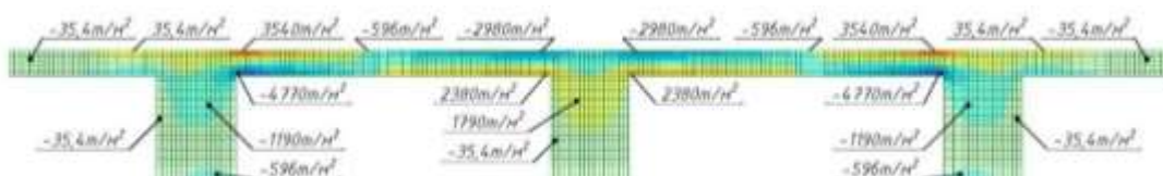
Рис. 9. Ізоліїнї нормальних напружень \sigma_{yy}
