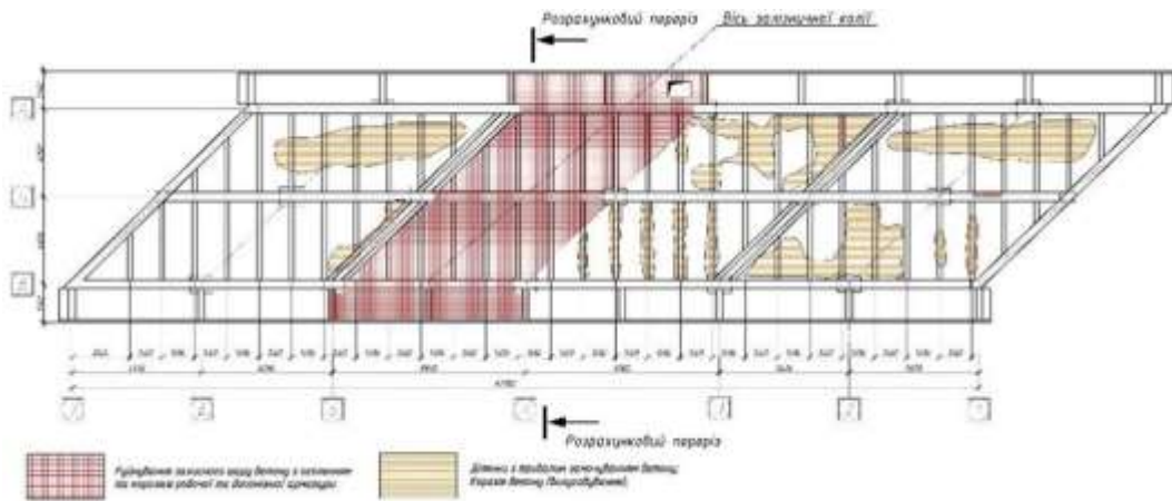
Рис. 3. План шляхопроводу з місцями найбільших руйнувань конструкцій по результатам обстеження [4]
