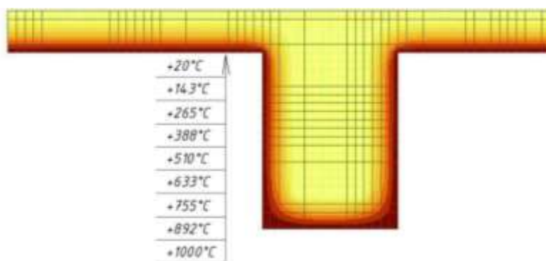
Рис. 6. Ізоліїнї температурних полів в фрагменті розрізу шляхопроводу
