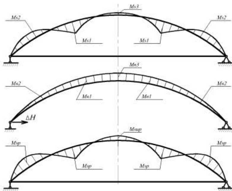
Рис. 8. Перерозподіл згинальних моментів в перерізах двохарнірної арки
