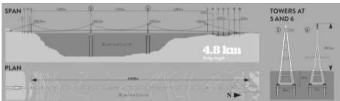
Рис. 21. Орієнтовний проект підвісного мосту [14]
