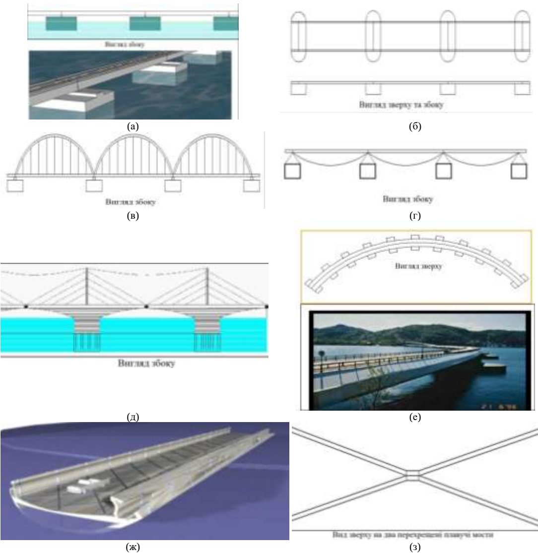
Рис. 11. Варіанти схем наплавного мосту SPFB [8]
