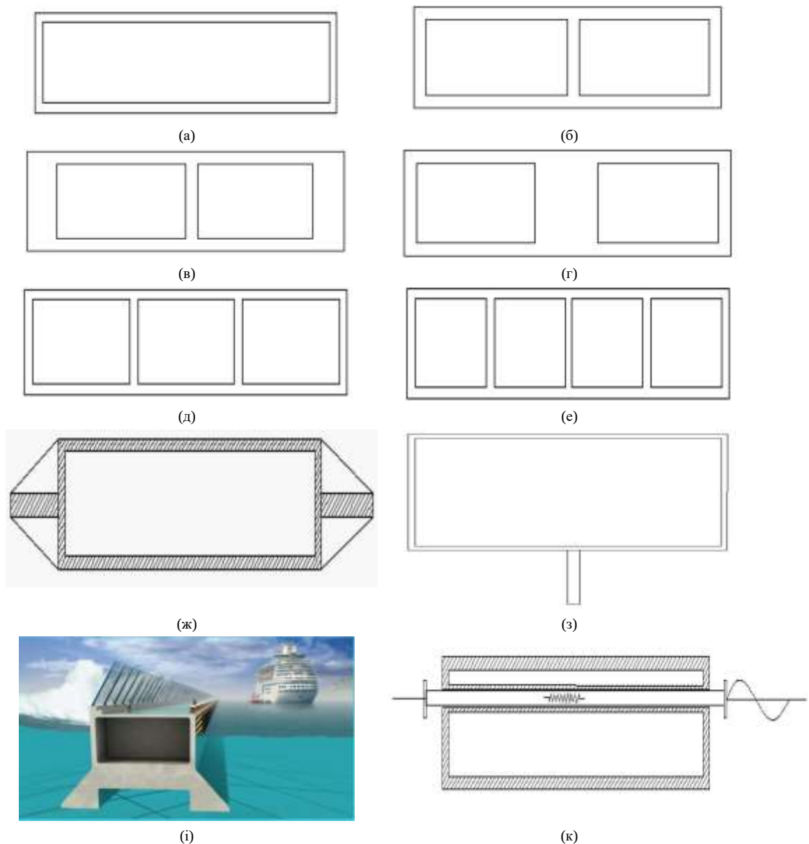
Рис. 12. Варіанти форми понтонів [8]
