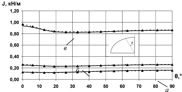
Рис. 5. Розподіл J-інтеграла вздовж фронту тріщини (суцільна лінія – пластична постановка; штрихова з трикутниками – пружна постановка) для напівеліптичних тріщин з розмірами напівосей: a – 0,5 та 0,3 мм; b – 0,63 та 0,47 мм; \sigma – 1,53 та 1,3 мм
