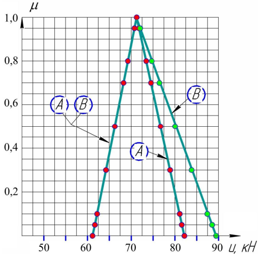
Рис. 5. Графічне зображення нечітких чисел \bar{u}_L(B) і \bar{u}_R(B)
