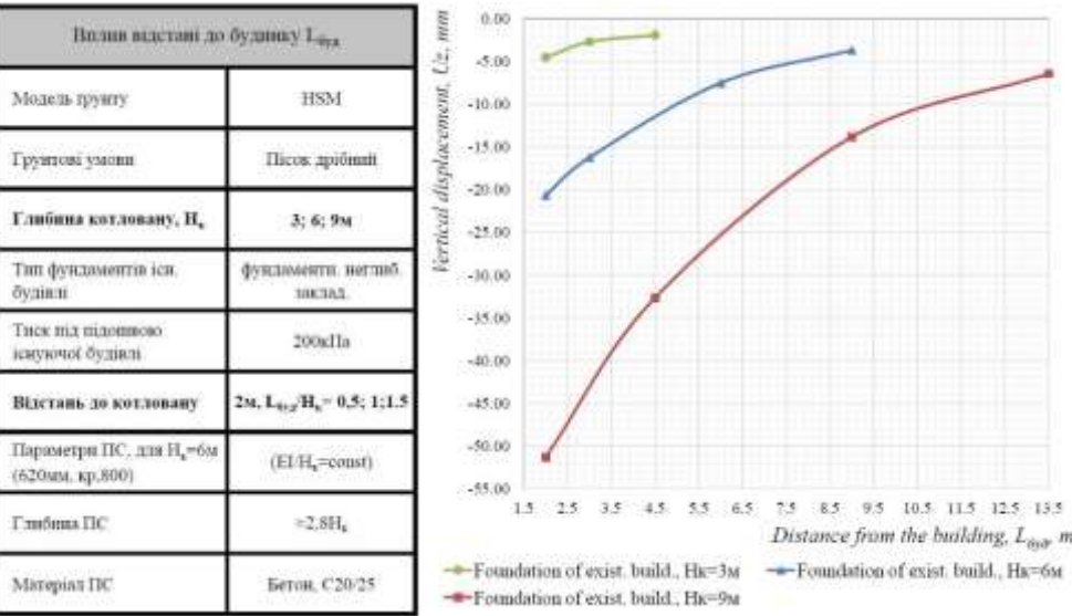
Рис. 6. Залежність додаткових осідань фундаменту існуючої будівлі від відстані до котловану L_{\text{буд}}
