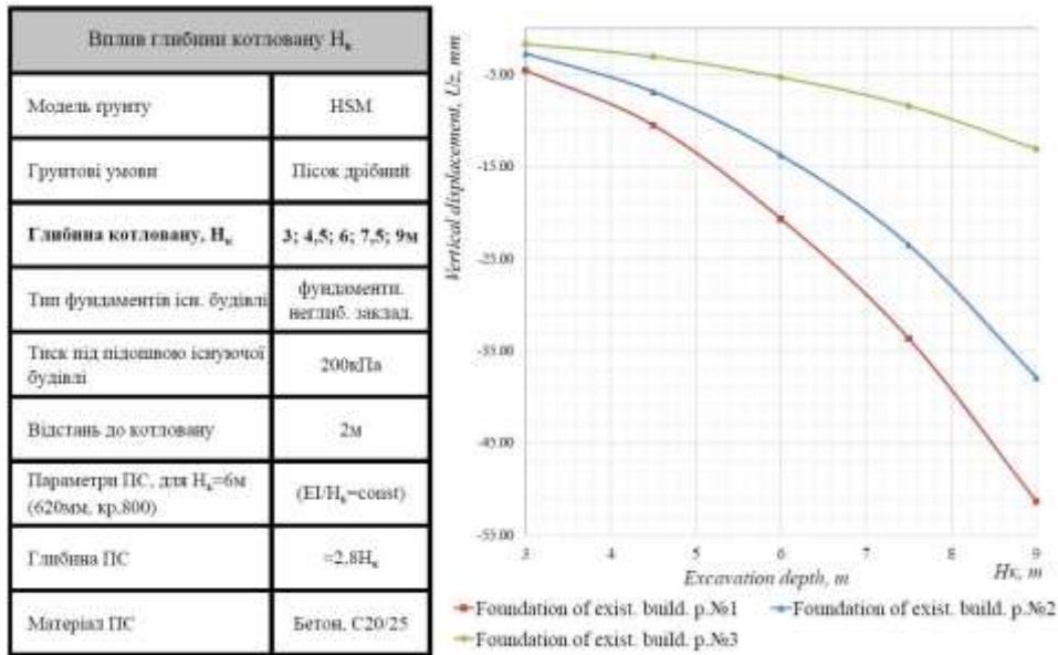
Рис. 5. Залежність додаткових осідань фундаменту існуючої будівлі від глибини котловану H_k
